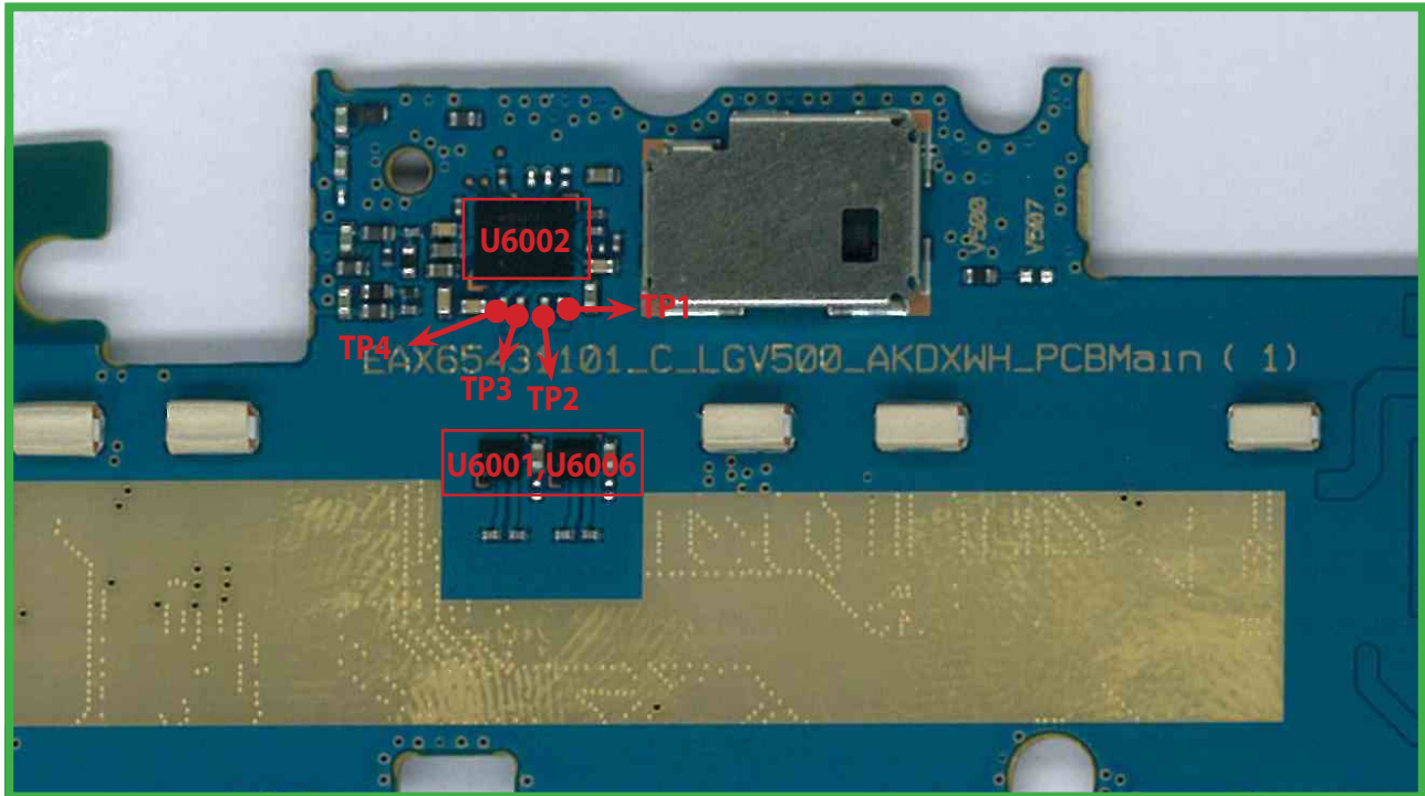
PCB TOP
