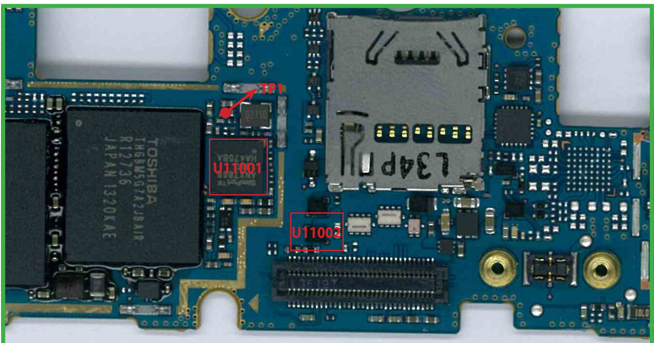
PCB Bottom
